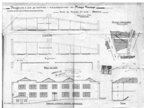
Fig. 4. Projeto das instalações da Fábrica de louça Esmaltada J. Minchin/Mário Navega na Rua do Freixo. Fonte: Licença de obras 1929/1263 .AHMP/CMP. F
